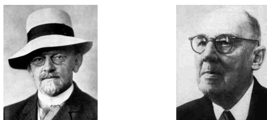
Fig. 3.21 David Hilbert 1862–1943 and Wacław Sierpiński, 1882–1969
