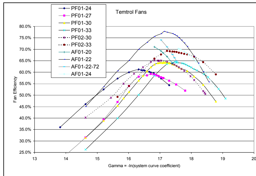
Figure 78. Temtrol Plenum Fan Data
