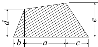
TRAPEZIUM
