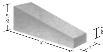
9 Inch Edge Skew 9 X (4½ – 1½) X 3
