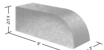
9 Inch Jamb 9 X 4½ X 3
