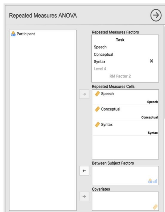
Figure 13-9 : Boîte de dialogue ANOVA pour mesures appariées avec Jamovi
