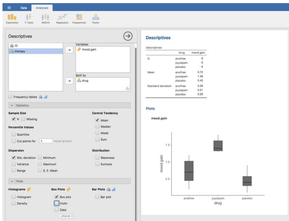
Figure 13-1 : Statistiques descriptive sur l'amélioration de l'humeur et diagrammes en boîtes par médicament administré
