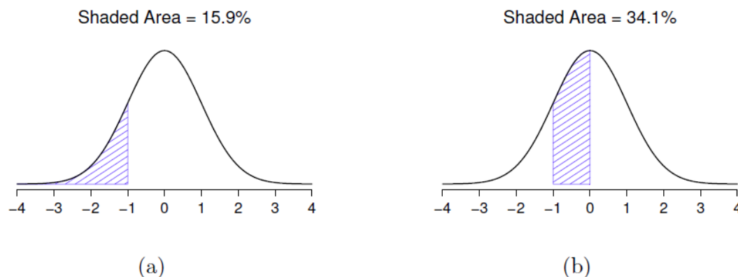
Figure 7-9 : Deux autres exemples de « l'aire sous l'idée de courbe ». Il y a 15,9 % de chances qu'une observation se situe un écart-type inférieur ou inférieur à la moyenne (panel a), et 34,1 % de chances que l'observation se situe quelque part entre un écart-type inférieur à la moyenne et la moyenne (panel b). Notez que si vous additionnez ces deux chiffres, vous obtenez 15,9\% + 34,1\% = 50\% . Pour les données normalement distribuées, il y a 50 % de chances qu'une observation soit inférieure à la moyenne. Et bien sûr, cela implique aussi qu'il y a 50 % de chances qu'elle soit supérieure à la moyenne.
