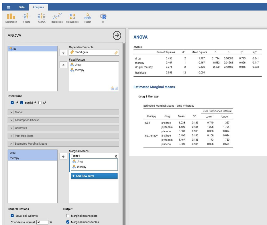
Figure 14-8 : capture d'écran de Jamovi montrant les moyennes marginales du modèle saturé, c'est-à-dire incluant la composante d'interaction, avec l'ensemble des données clinicaltrial
