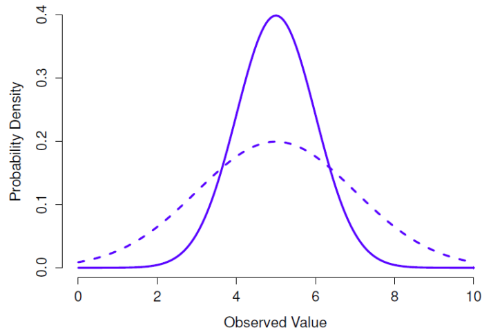
Figure 7-7 : Une illustration de ce qui se passe lorsque vous modifiez l'écart-type d'une distribution normale. Les deux distributions représentées dans cette figure ont une moyenne de \mu = 5 , mais elles ont des écarts-types différents. La ligne pleine correspond à une distribution avec un écart-type \sigma = 1 , et la ligne pointillée montre une distribution avec un écart-type \sigma = 2 . Par conséquent, les deux distributions sont « centrées » au même endroit, mais la ligne pointillée est plus large que la solide.
