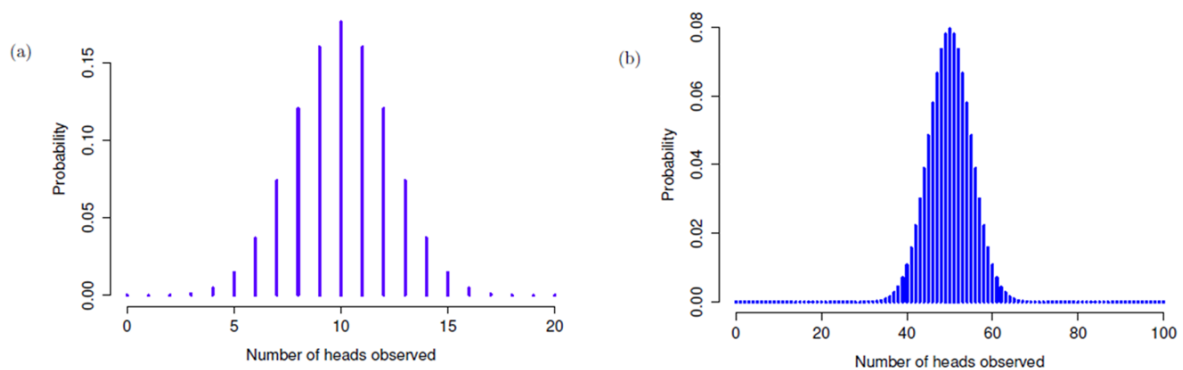
Figure 7-4 : Deux distributions binomiales, impliquant un scénario dans lequel je tire à pile ou face, donc la probabilité de succès sous-jacente est \theta = 1/2 . Dans le graphique (a), nous supposons que je lance la pièce N = 20 fois. Dans le panneau (b) nous supposons que la pièce est lancée N = 100 fois.
