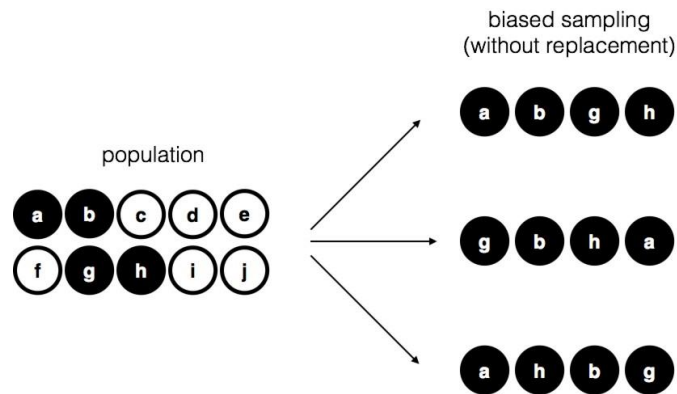
Figure 8-2 : Échantillonnage biaisé sans remplacement à partir d'une population finie
