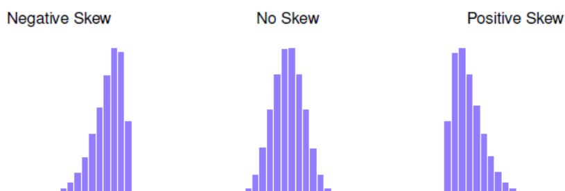
Figure 4-11 : Une illustration de l'asymétrie (skew). Sur la gauche nous avons un ensemble de données négatives ( skewness = -.93 ), au milieu nous avons un ensemble de données sans asymétrie (enfin, presque pas : skewness = -.006 ), et sur la droite nous avons un ensemble de données positivement asymétriques ( skewness = .93 ).
