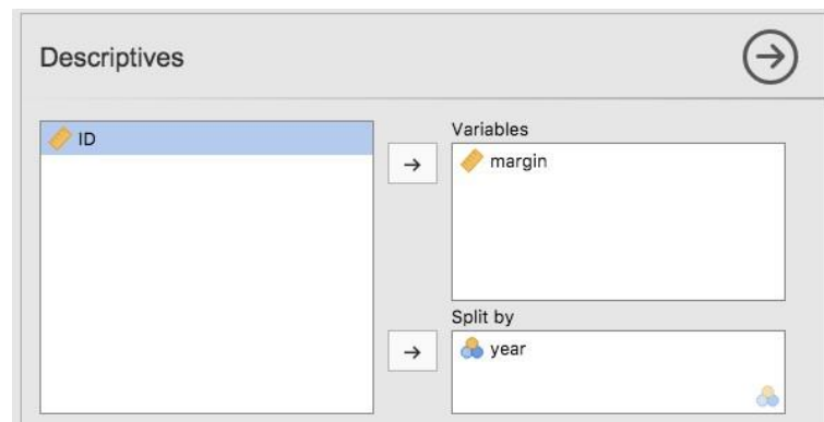
Figure 5-6 : Capture d'écran de Jamovi montrant la fenêtre « Split by »
