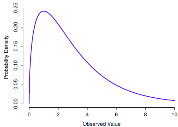
Figure 7-11 : Une distribution \chi^2 avec 3 degrés de liberté. Notez que les valeurs observées doivent toujours être supérieures à zéro et que la distribution est assez asymétrique. Ce sont les principales caractéristiques d'une distribution du chi carré
