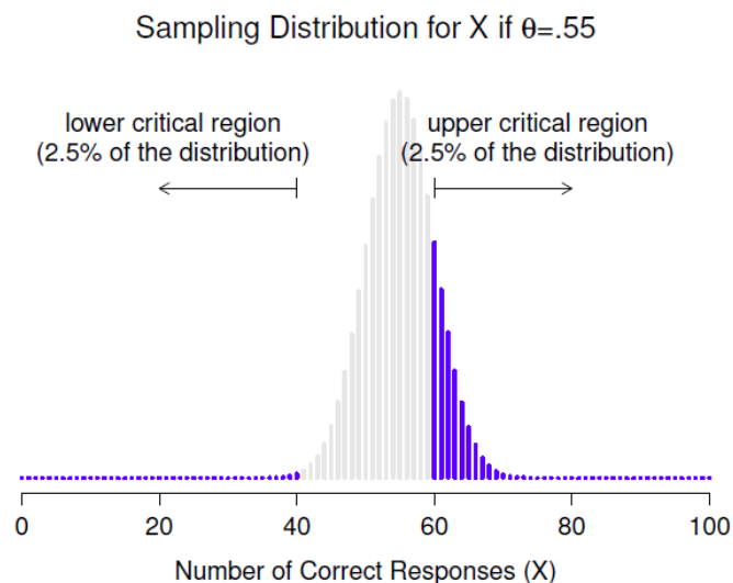
Figure 9-5 : Distribution de l'échantillonnage sous l'hypothèse alternative pour une valeur de paramètre de population de \theta = 0.55 . Une proportion raisonnable de la distribution se trouve dans la région de rejet.
