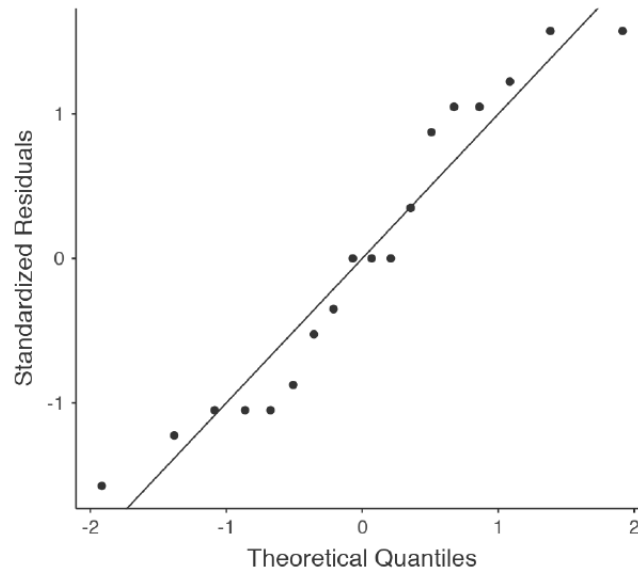
Figure 14-10 : Vérification des présupposés dans un modèle d'ANOVA
