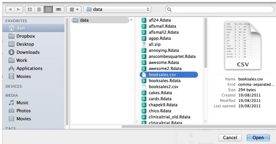
Figure 3-4: Une boîte de dialogue sur un Mac vous demandant de sélectionner le fichier csv que Jamovi devrait essayer d'importer. Les utilisateurs de Mac le reconnaîtront immédiatement, c'est la manière habituelle dont un Mac vous demande de trouver un fichier. Les utilisateurs de Windows ne verront pas cela, au lieu de cela, ils verront la fenêtre habituelle de l'explorateur que Windows vous donne toujours quand il veut que vous sélectionniez un fichier.
