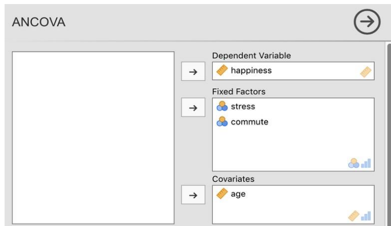
Figure 14-12 : La fenêtre d'analyse ANCOVA de Jamovi
