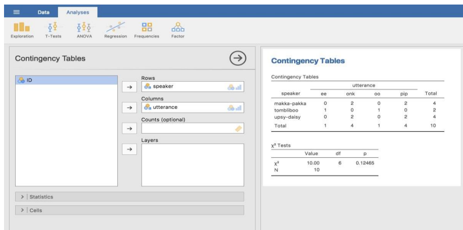
Figure 6-2 : Tableau de contingence pour le locuteur et les variables des énoncés
