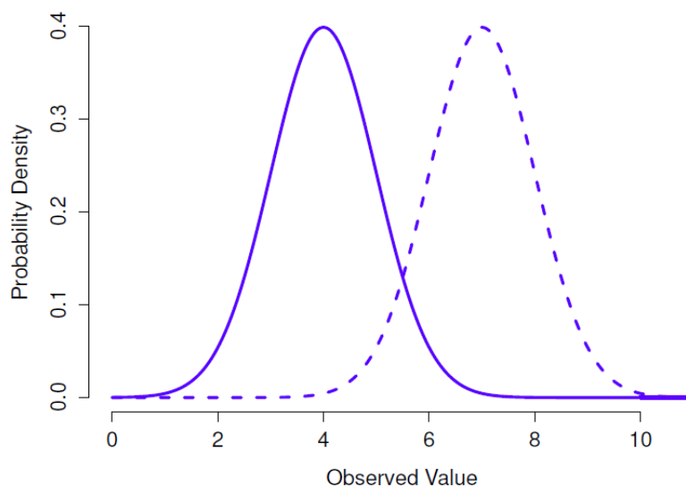
Figure 7-6 : Une illustration de ce qui se passe lorsque vous modifiez la moyenne d'une distribution normale. Dans les deux cas, l'écart-type est \sigma = 1 . Comme on pouvait s'y attendre, les deux distributions ont la même forme, mais la ligne en pointillés est décalée vers la droite.
