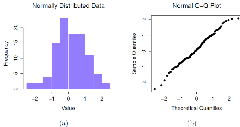
Figure 11-20 : Histogramme (figure a) et graphique QQ normal (figure b) de données normales , un échantillon normalement distribué avec 100 observations. La statistique Shapiro-Wilk associée à ces données est W = .99 , ce qui indique qu'aucun écart significatif par rapport à la normalité n'a été détecté ( p = .73 )
