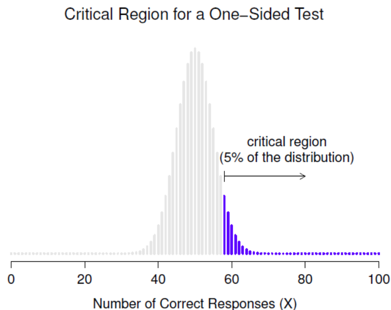
Figure 9-3 : La région critique pour un essai unilatéral. Dans ce cas, l'hypothèse alternative est que \theta > .5 de sorte que nous ne rejeterions que l'hypothèse nulle pour les grandes valeurs de X . Par conséquent, la région critique ne couvre que la partie supérieure de la queue de la distribution d'échantillonnage, en particulier les 5 % supérieurs de la distribution. Comparez cela à la version bilatérale de la figure 9.2.
