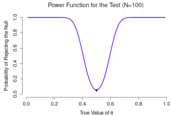
Figure 9-7 : La probabilité que nous rejeterons l'hypothèse nulle, tracée en fonction de la valeur réelle de \vartheta . Évidemment, le test est plus puissant (plus grande chance de rejet correct) si la valeur réelle de \theta est très différente de la valeur spécifiée dans l'hypothèse nulle (i.e. \theta = .5 ). Notez que lorsque \theta est en fait égal à .5 (représenté par un point noir), l'hypothèse nulle est en fait vraie et rejeter l'hypothèse nulle dans ce cas serait une erreur de type I.
