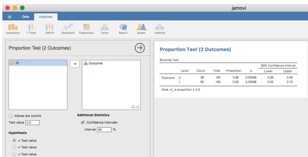
Figure 9-4 : Analyse du test binomial et résultats dans Jamovi
