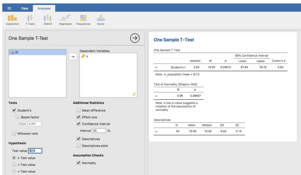
Figure 11-6 : Jamovi effectue le test t sur un échantillon.
