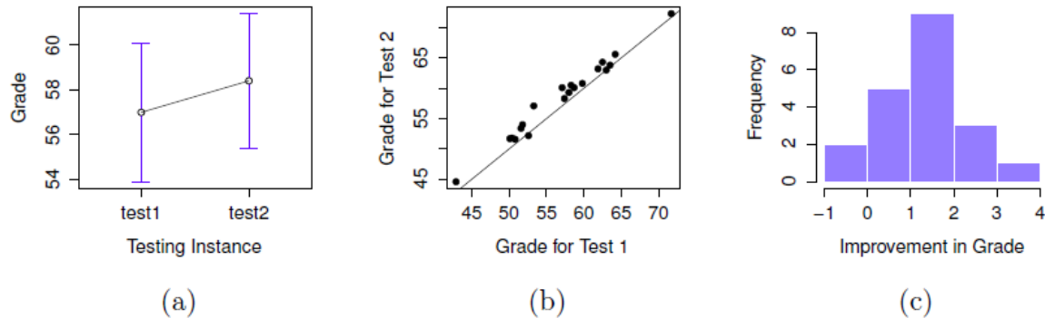
Figure 11-14 : Note moyenne pour l'essai 1 et l'essai 2, avec des intervalles de confiance associés à 95 % (panel a). Diagramme de dispersion montrant les notes individuelles pour l'essai 1 et l'essai 2 (panneau b). Histogramme montrant l'amélioration réalisée par chaque élève de la classe du Dr Chico (panel c). Dans le panneau c, remarquez que la distribution est presque entièrement au-dessus de zéro : la grande majorité des élèves ont amélioré leur performance du premier au deuxième test.
