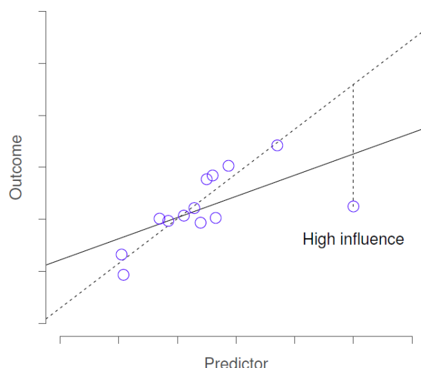
Figure 12-19 : Illustration des points d'influence élevés. Dans ce cas, l'observation anormale est très inhabituelle sur la variable prédictive (axe des x) et se situe très loin de la ligne de régression. Par conséquent, la ligne de régression est fortement déformée, même si (dans ce cas) l'observation anormale est tout à fait typique en termes de variable résultat (axe des y).
