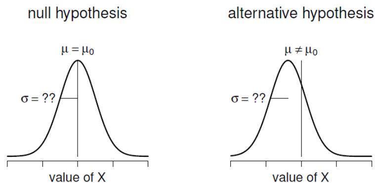
Figure 11-4 : Illustration graphique de l'hypothèse nulle et de l'hypothèse alternative supposée par le test t pour un échantillon (bilatéral). Notez la similitude avec le test z (Figure 11-2). L'hypothèse nulle est que la moyenne de population \mu est égale à une valeur spécifiée \mu_0 , et l'hypothèse alternative est que ce n'est pas le cas. Comme pour le test z, nous supposons que les données sont normalement distribuées, mais nous ne supposons pas que l'écart type de population \sigma est connu à l'avance.
