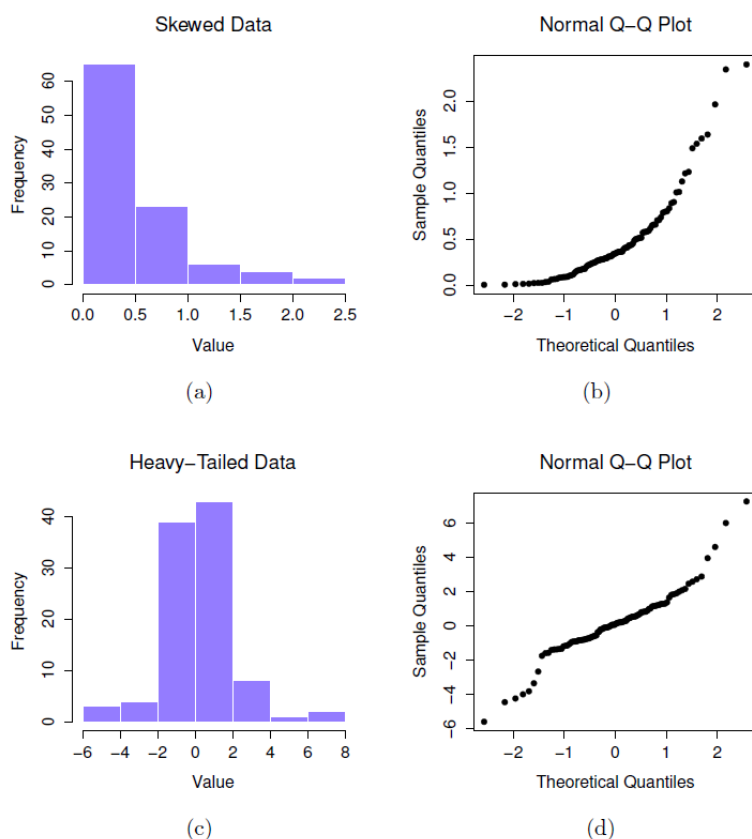
Figure 11-21 : Dans la rangée du haut, un histogramme (figure a) et un graphique QQ normal (figure b) des 100 observations d'un ensemble de données skewed.data . L'asymétrie des données ici est de 1,94 et se reflète dans un graphique QQ qui s'incurve vers le haut. En conséquence, la statistique de Shapiro-Wilk est W = .80 , ce qui reflète un écart important par rapport à la normalité ( p < .001 ). La rangée du bas montre les mêmes graphiques pour un ensemble de données à queues pointues, qui se compose de 100 observations. Dans ce cas, les queues pointues dans les données produisent une kurtosis élevée (2,80), et provoquent l'aplatissement de la courbe QQ au milieu, et une forte courbe de chaque côté. La statistique Shapiro-Wilk résultante est W = .93 , ce qui reflète une fois de plus une non-normalité importante ( p < .001 ).
