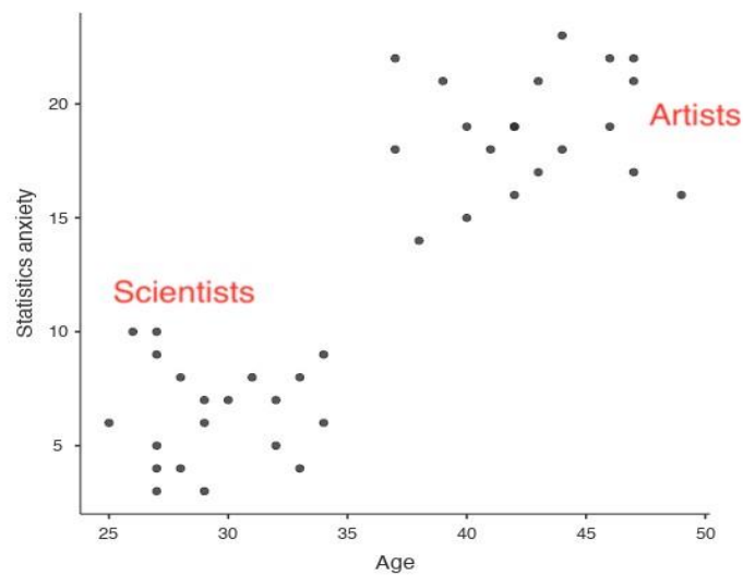
Figure 14-11 : Représentation graphique de l'aversion aux statistiques par rapport à l'âge pour deux groupes distincts
