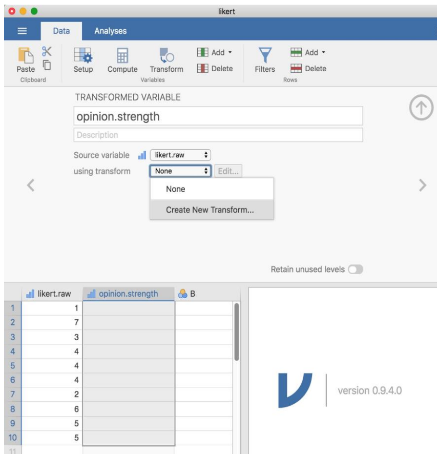
Figure 6-8 : Création d'une nouvelle transformation de variable à l'aide de la commande Jamovi « Transform ».
