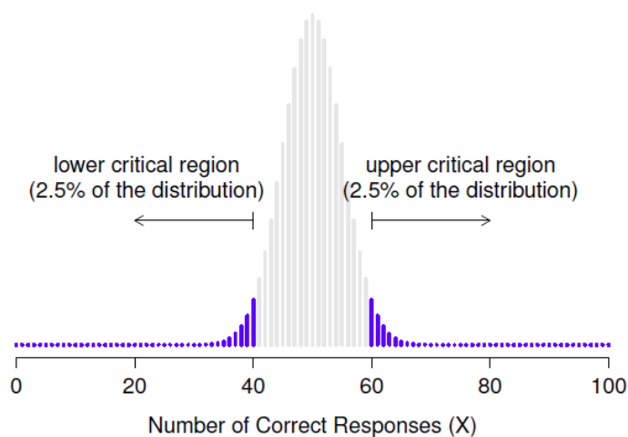
Figure 9-2 : La région critique associée au test d'hypothèse pour l'étude ESP, pour un test d'hypothèse avec un niveau de signification de \alpha = .05 . Le graphique montre la distribution d'échantillonnage de X sous l'hypothèse nulle (c.-à-d. identique à la Figure 9-1). Les barres grises correspondent aux valeurs de X pour lesquelles on retiendrait l'hypothèse nulle. Les barres bleues (plus foncées) indiquent la région critique, ces valeurs de X pour lesquelles nous rejeterions la valeur nulle. Étant donné que l'hypothèse alternative est bilatérale (c.-à-d. qu'elle permet à la fois \theta < .5 et \theta > .5 ), la région critique couvre les deux queues de la distribution. Pour assurer un niveau de .05 à \alpha , nous devons nous assurer que chacune des deux régions englobe 2,5 % de la distribution de l'échantillonnage.
