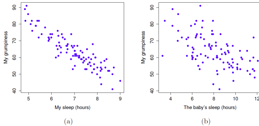
Figure 12-2 : Diagrammes de dispersion montrant la relation entre dan.sleep et dan.grump (à gauche) et la relation entre baby.sleep et dan.grump (à droite)
