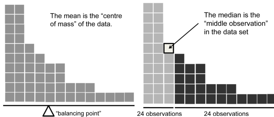
Figure 4-4 : Une illustration de la différence entre l'interprétation de la moyenne et celle de la médiane. La moyenne est essentiellement le « centre de gravité » de l'ensemble de données. Si vous imaginez que l'histogramme des données est un objet solide, alors le point sur lequel vous pouvez l'équilibrer (comme sur une bascule) est la moyenne. Par contre, la médiane est l'observation du milieu, la moitié des observations étant plus petites et la moitié plus grandes.
