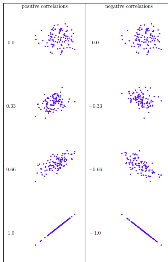
Figure 12-4 : Illustration de l'effet de la variation de l'intensité et de la direction d'une corrélation. Dans la colonne de gauche, les corrélations sont 0 ; 0,33 ; 0,66 et 1 ; dans la colonne de droite, les corrélations sont 0, -0,33, -0,66 et -1.
