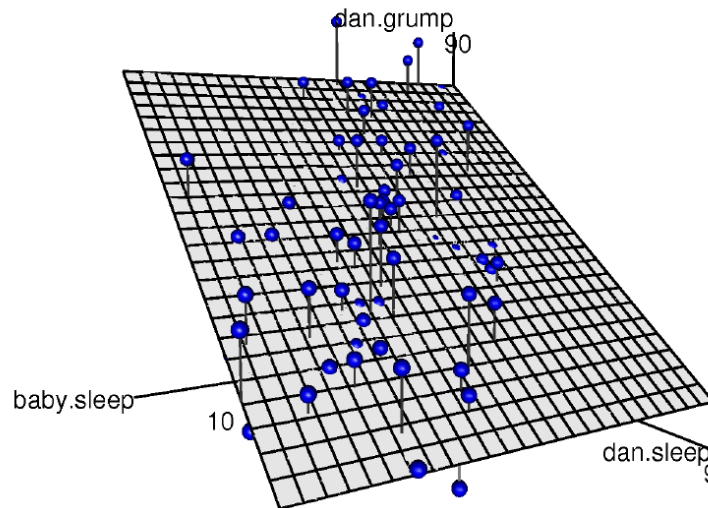
Figure 12-14 : Visualisation 3D d'un modèle de régression multiple. Il y a deux prédicteurs dans le modèle, dan.sleep et baby.sleep , et la variable de résultat est dan.grump . Ensemble, ces trois variables forment un espace 3D. Chaque observation (point) est un point dans cet espace. De la même manière qu'un modèle de régression linéaire simple forme une ligne dans un espace 2D, ce modèle de régression multiple forme un plan dans un espace 3D. Lorsque nous estimons les coefficients de régression, nous essayons de trouver un plan aussi proche que possible de tous les points bleus.
