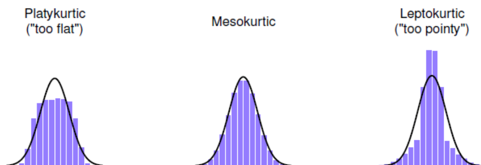
Figure 4-12: Une illustration de l'aplatissement. À gauche, nous avons un ensemble de données « platykurtique » (kurtosis = -0.95) qui signifie que l'ensemble de données est « trop plat ». Au milieu, nous avons un ensemble de données « mésokurtiques » (kurtosis est presque égal à 0), ce qui signifie que la précision des données est à peu près correcte. Enfin, à droite, nous avons un ensemble de données « leptokurtiques » (kurtosis = 2.12) indiquant que l'ensemble de données est « trop pointu ». Notez que l'aplatissement est mesuré par rapport à une courbe normale (ligne noire).
