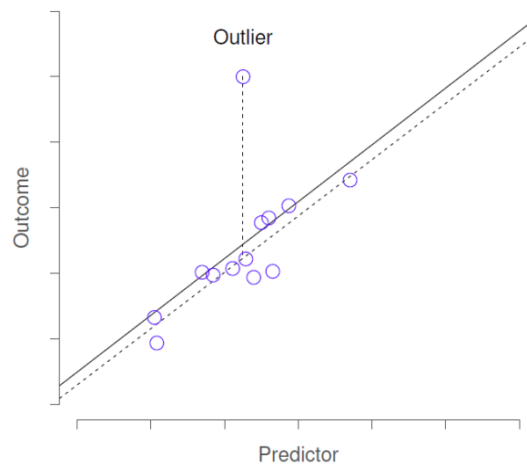
Figure 12-17 : Une illustration des valeurs aberrantes. Les lignes pointillées représentent la ligne de régression qui aurait été estimée sans l'observation anormale incluse, et le résidu correspondant (c.-à-d. le résidu de Studentisé). La ligne continue montre la ligne de régression avec l'observation anormale incluse. La valeur aberrante a une valeur inhabituelle sur la variable résultat (emplacement de l'axe des y), mais pas sur le prédicteur (emplacement de l'axe des x), et se trouve loin de la ligne de régression.
