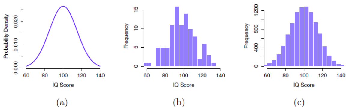
Figure 8-4 : La distribution de la population des scores de QI (panel a) et deux échantillons tirés au hasard. Dans le panel b, nous avons un échantillon de 100 observations, et dans le panel c, nous avons un échantillon de 10 000 observations.
