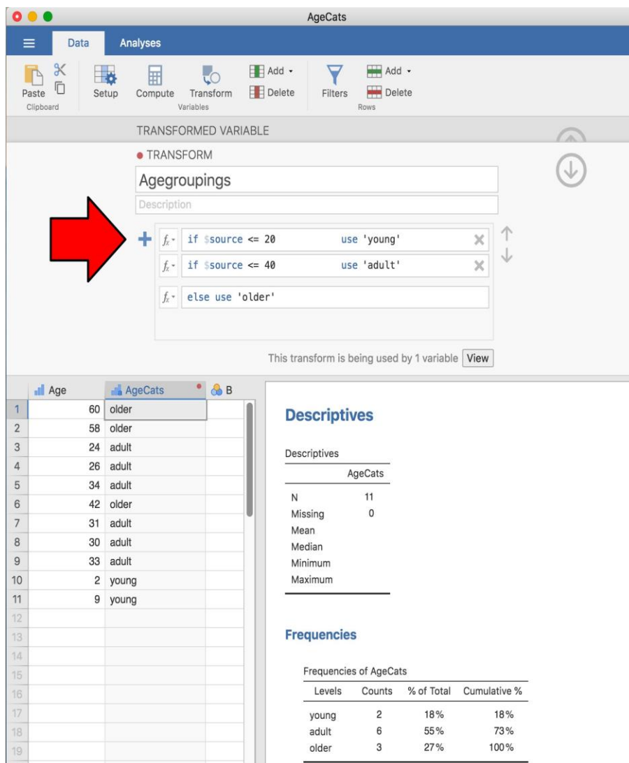
Figure 6-10 : Transformation de Jamovi en trois catégories d'âge, à l'aide du bouton 'Ajouter condition'.
