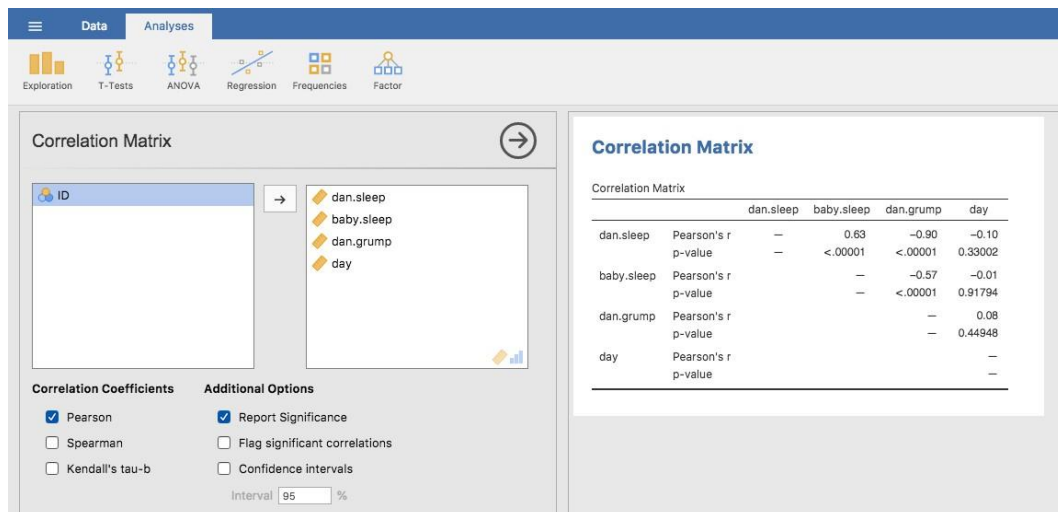
Figure 12-5 : Une capture d'écran Jamovi montrant les corrélations entre les variables du fichier parenthood.csv
