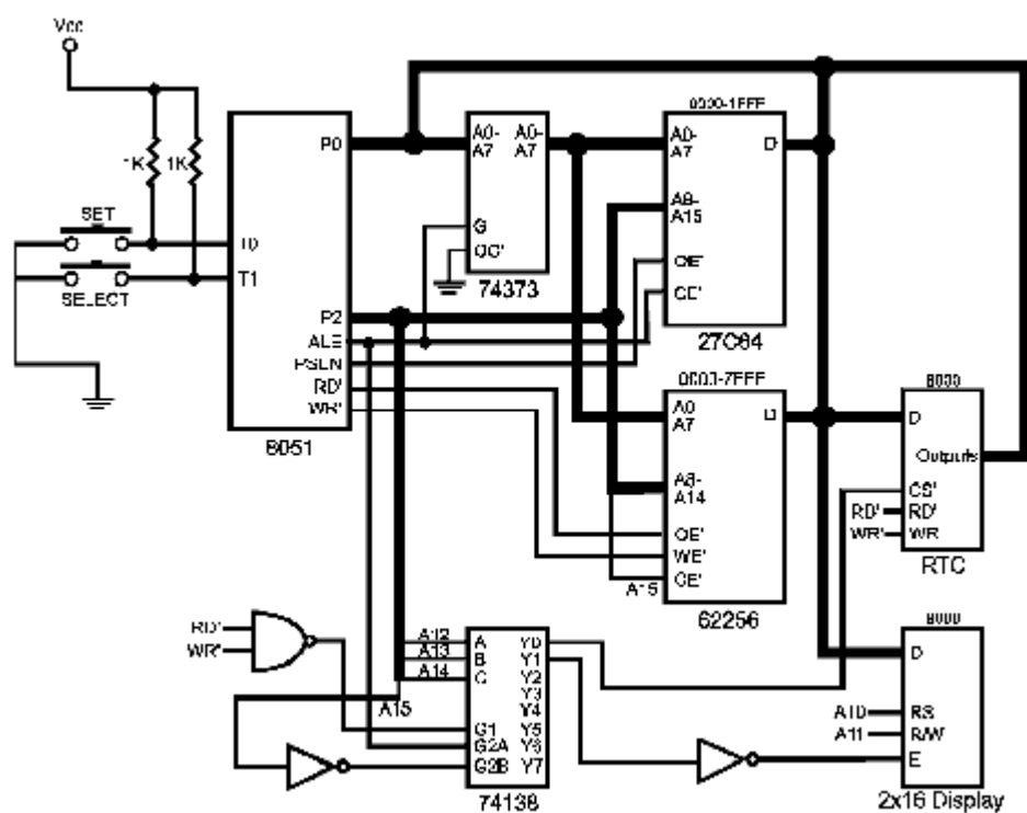
图 0-2 扩展电路
