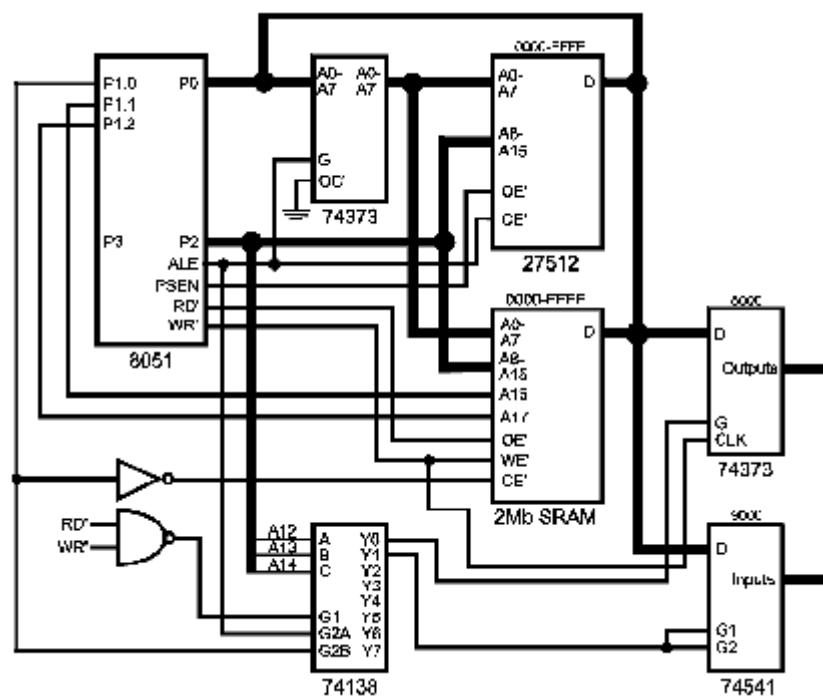
图0-4 页寻址RAM
