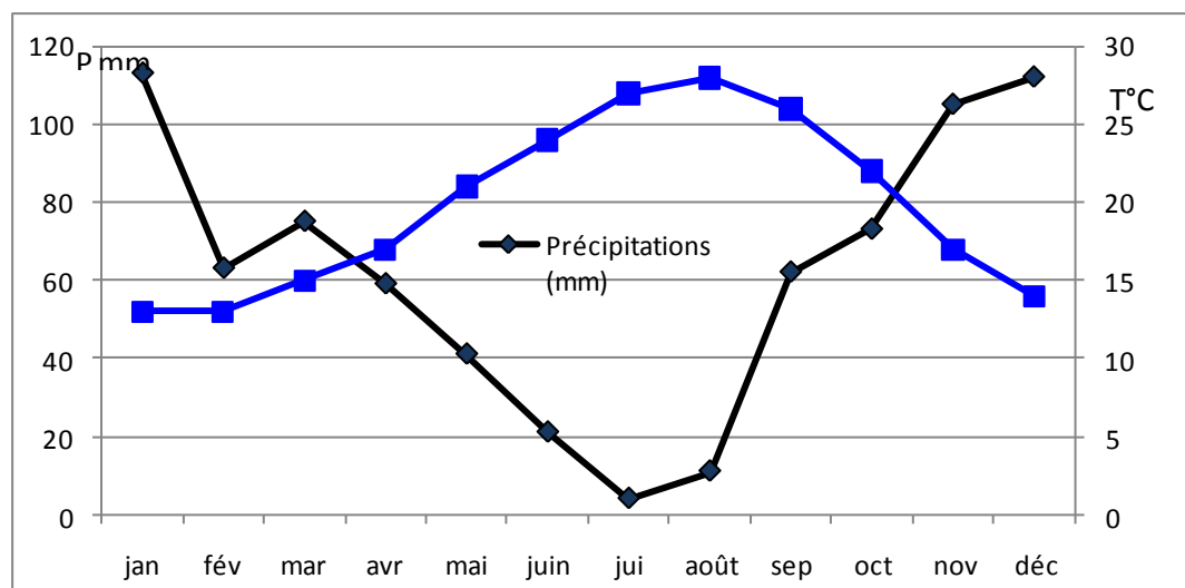
Figure 8 : Exemple de diagramme ombrothermique de Gaussen
