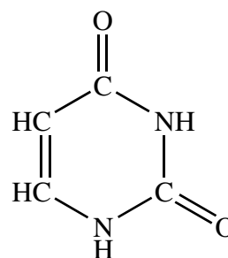
Uracil (U)
