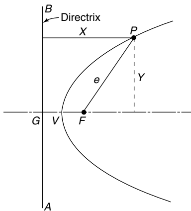
FIGURE A.2. Parabola.
