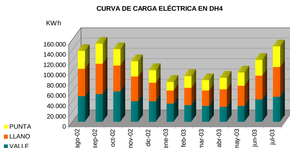
Figura 5. Consumos eléctricos mensuales según períodos.
