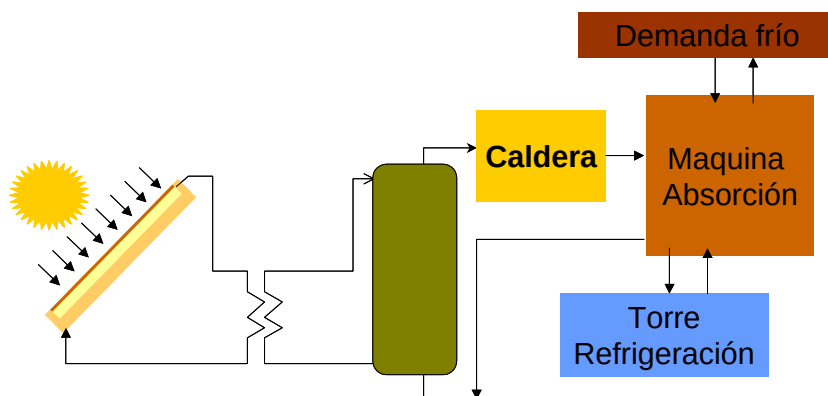
Figura 8. Esquema tipo de aplicación solar para refrigeración sólo con máquina de absorción.
