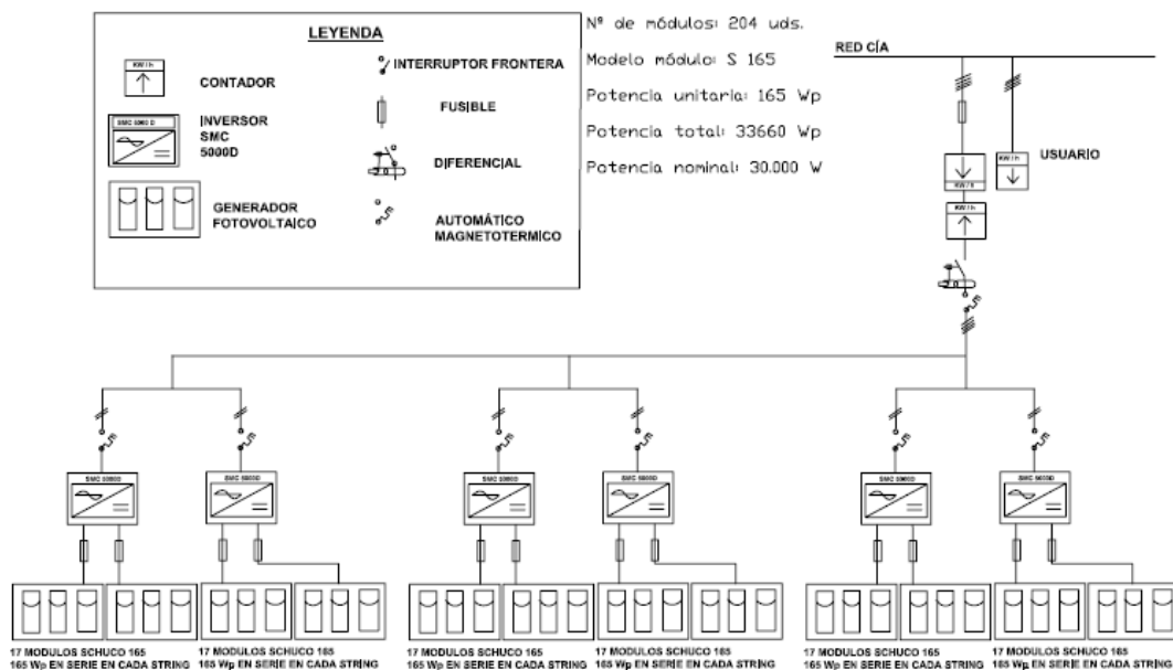
Figura 6. Esquema eléctrico de la piscina de La Unión.
