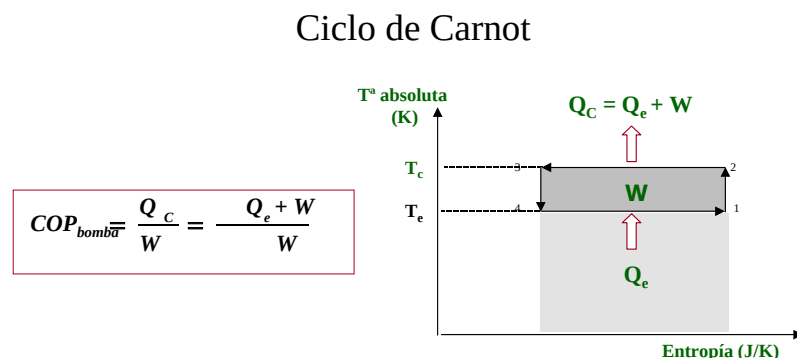
Figura 2. Ciclo bomba de calor.
