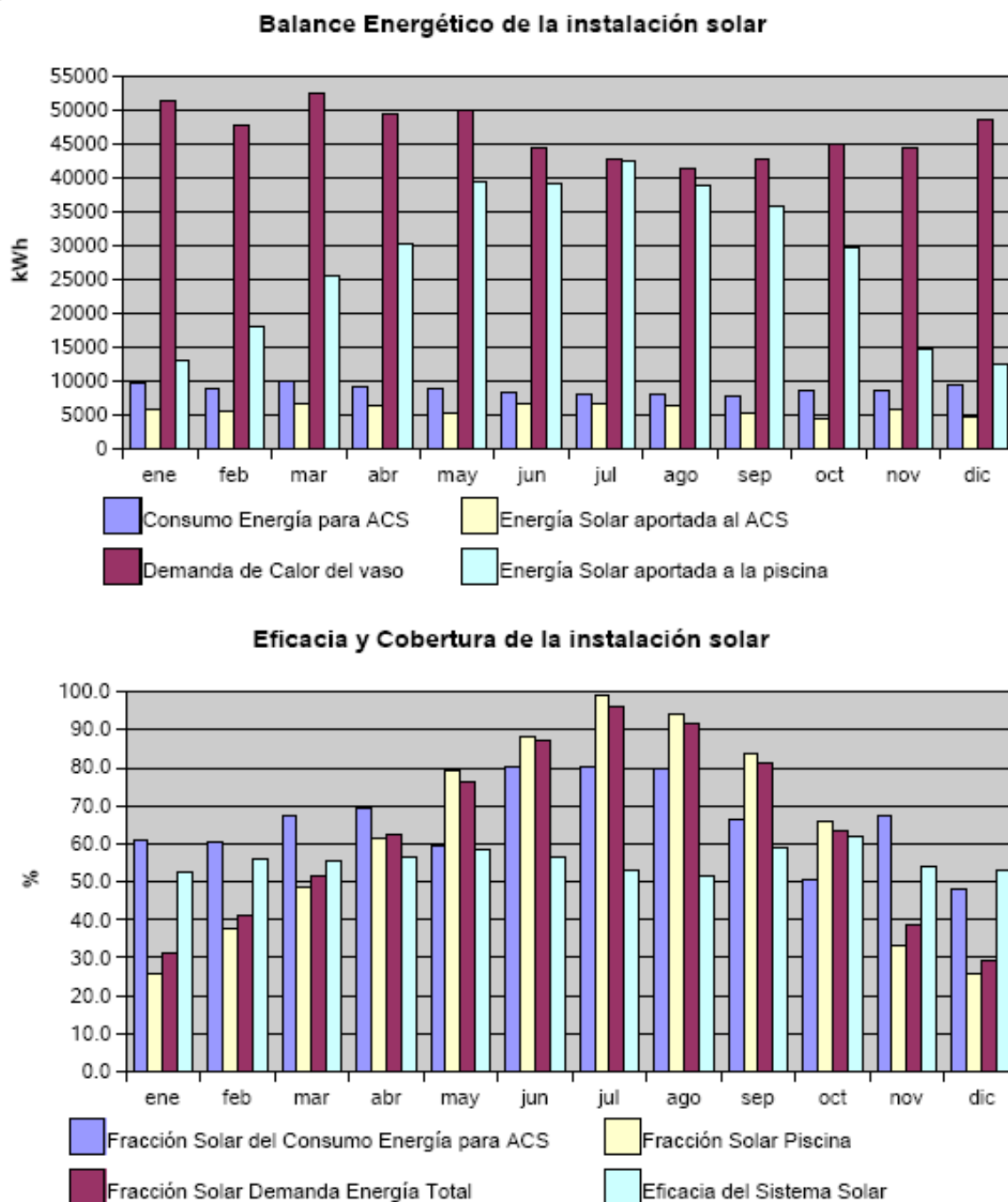
Figura 10. Gráficos del balance energético y de la eficacia y cobertura de la instalación solar. Polideportivo en Boadilla.
