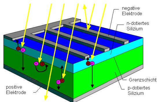
Figura 1. Sección de célula fotovoltaica.
