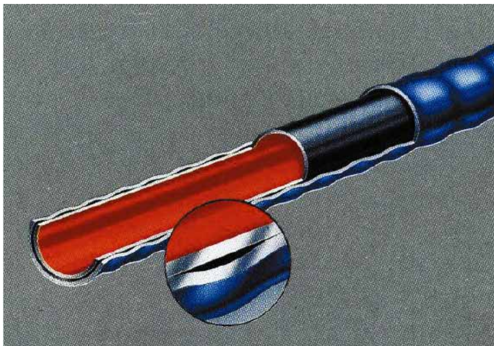
Figura 3. Tubo Duplex de la caldera Vitomax 300.
