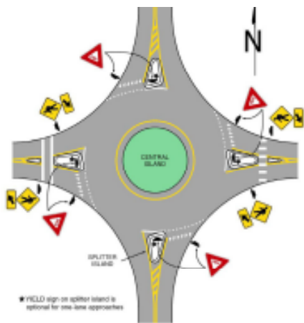
Mini Roundabout
